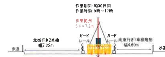
道路中央分離帯の作業状況図
