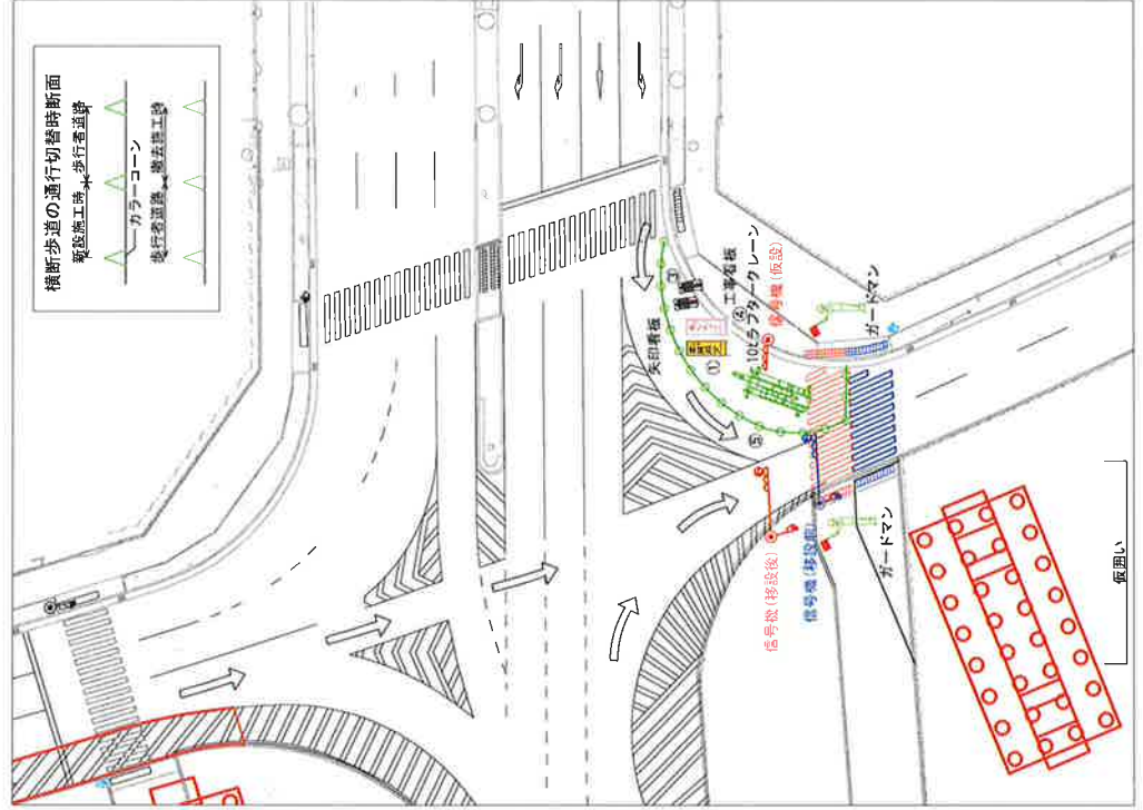
② 南面施工時
