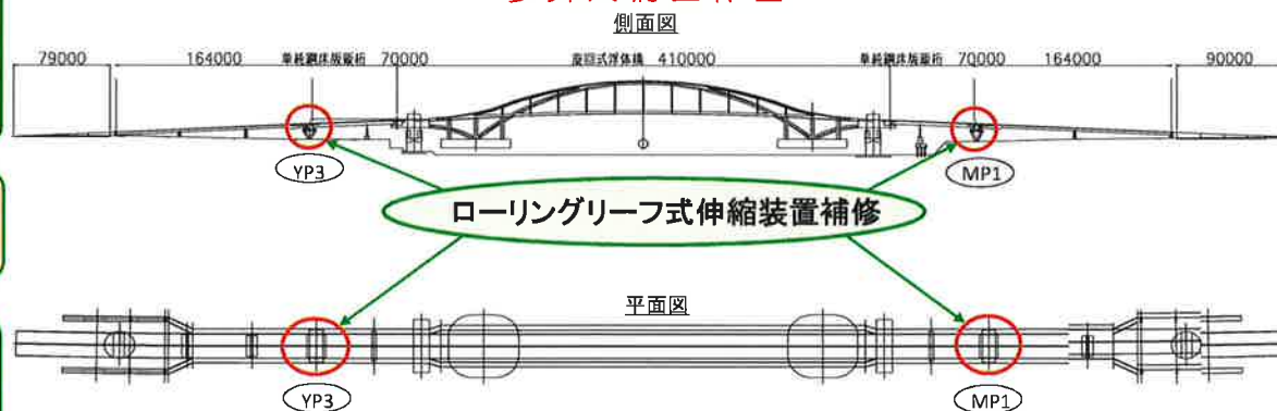
夢舞大橋全体図
