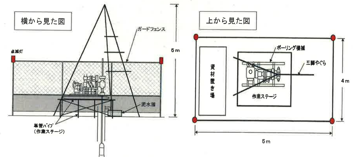
やぐら足場配置図
