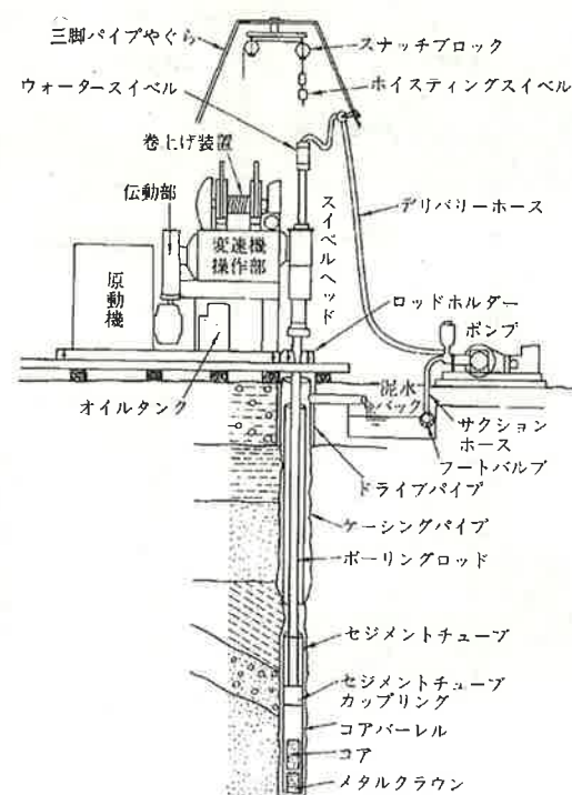
ボーリング模式図
