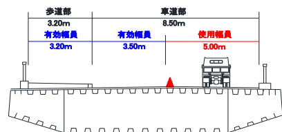
交通規制時断面【①施工範囲L=280m、②施工範囲L=280m】 交通規制時断面【③施工範囲L=280m、④施工範囲L=280m】
