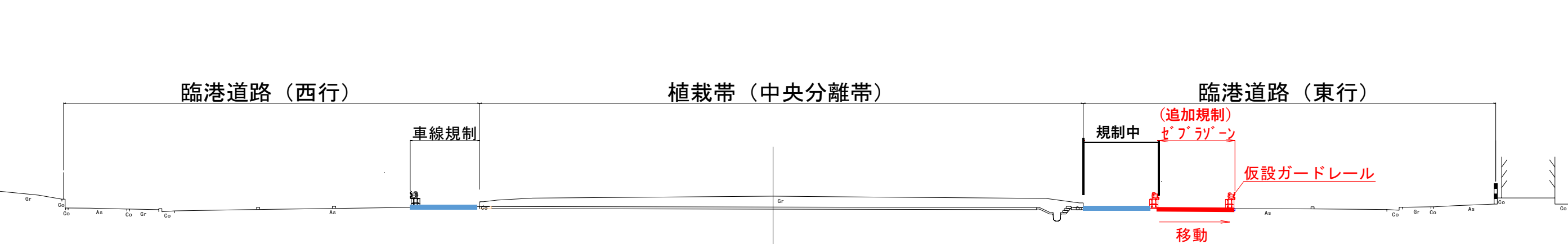
追加規制断面図
