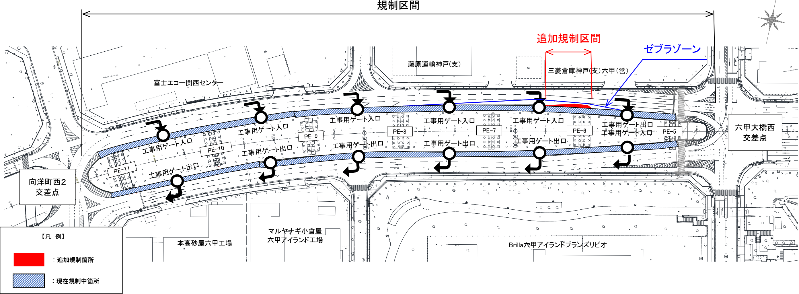
追加規制平面図
