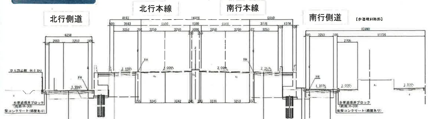
切替後断面図
