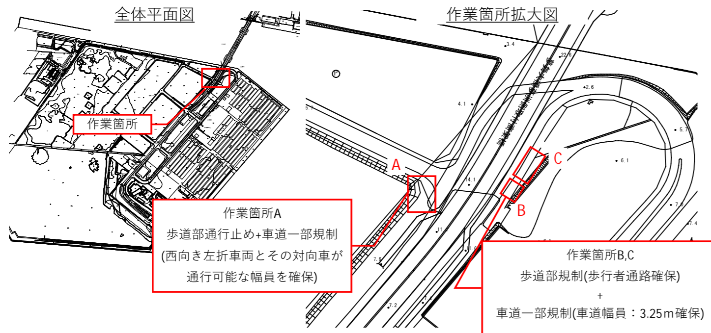
作業箇所平面図
