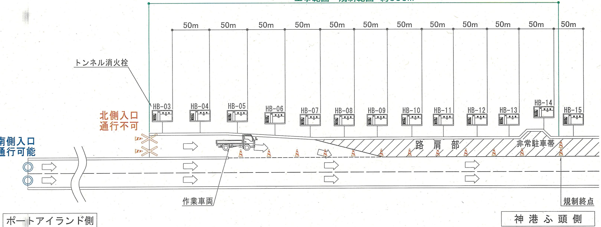
工事範囲＝規制範囲 約600m
