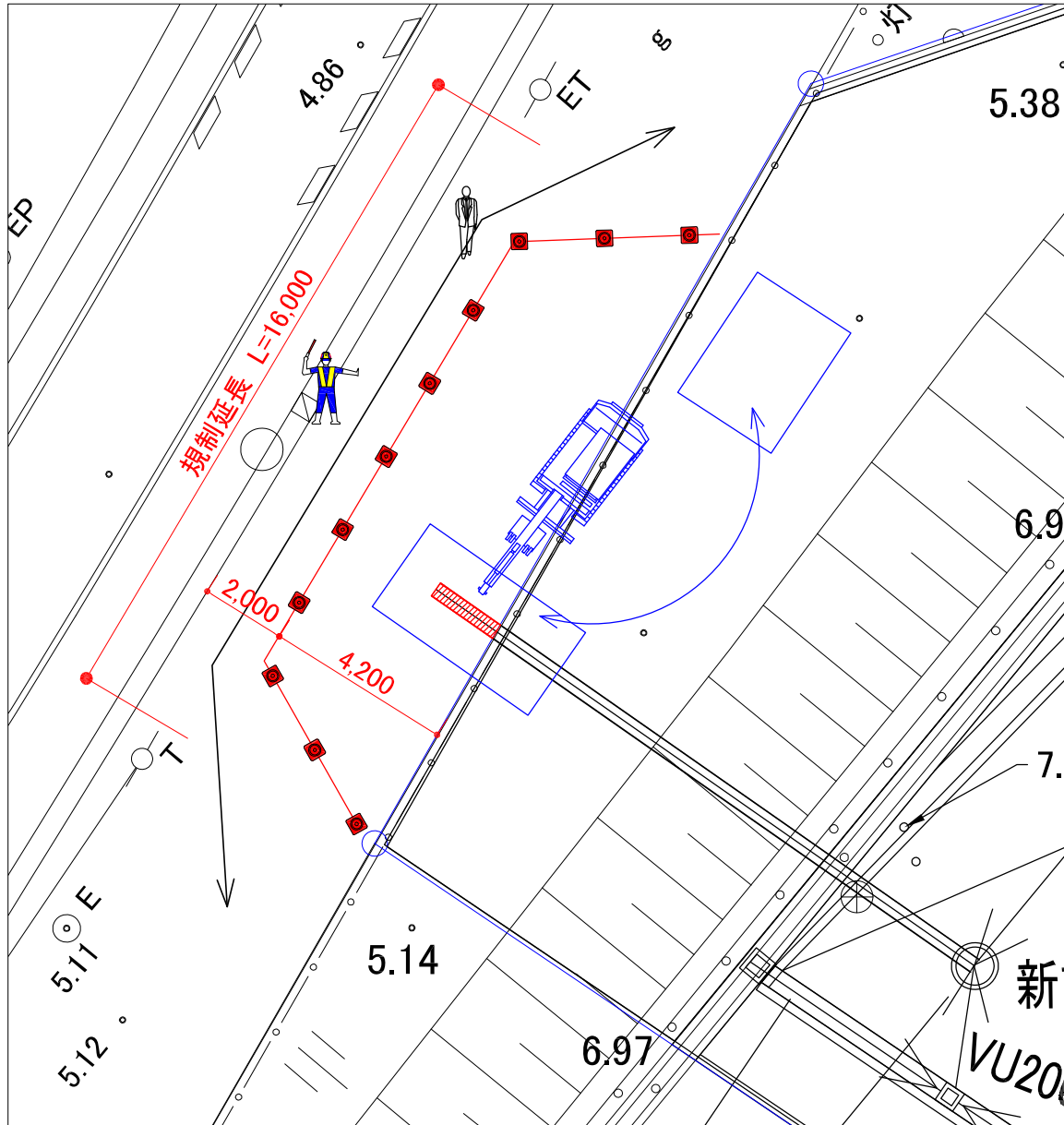
平面图
